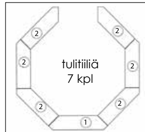
1. kerros tulitiiliä
